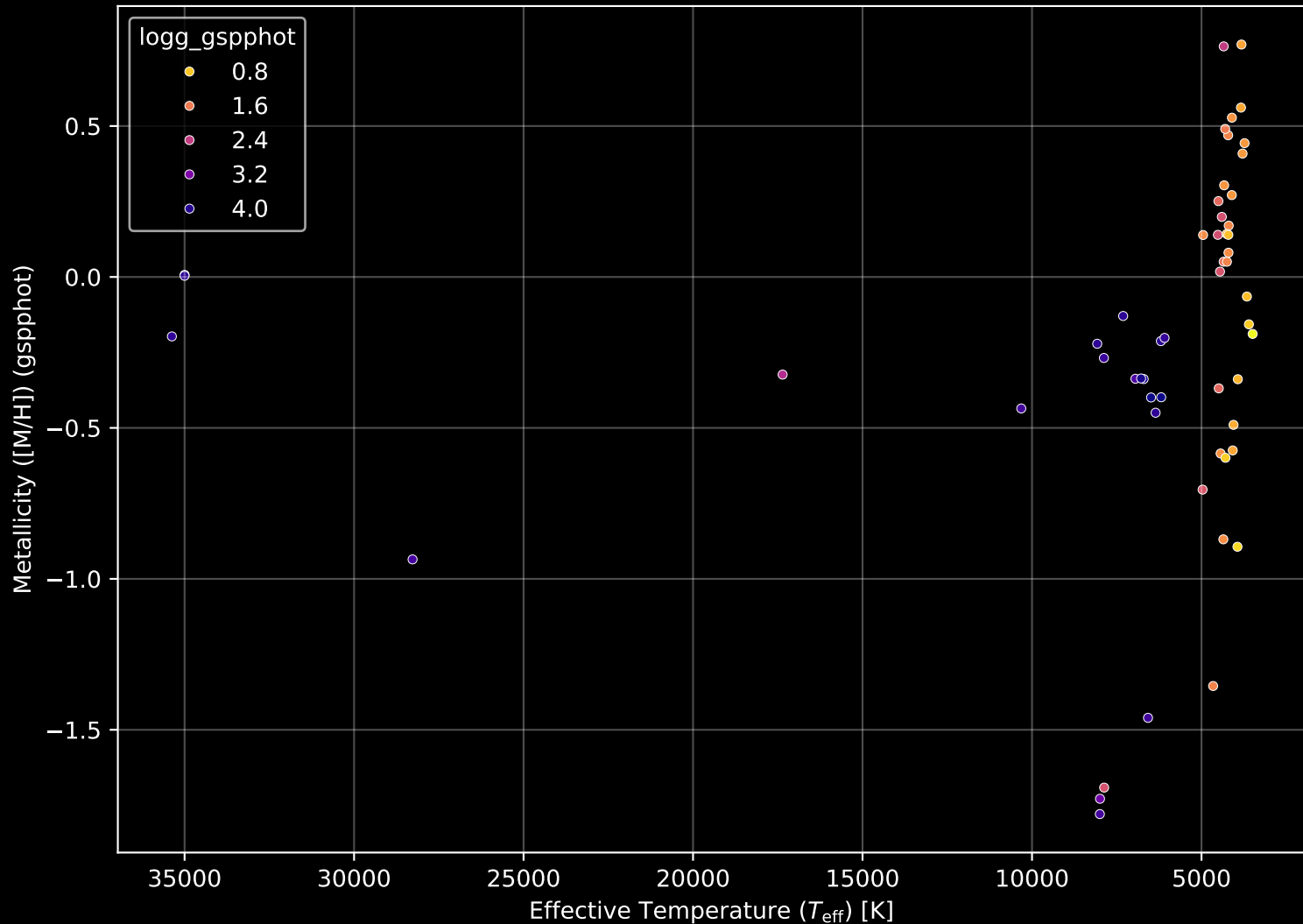
APOGEE DR17 Field: [282-32-O] Stellar Population Parameters (n= 55)
