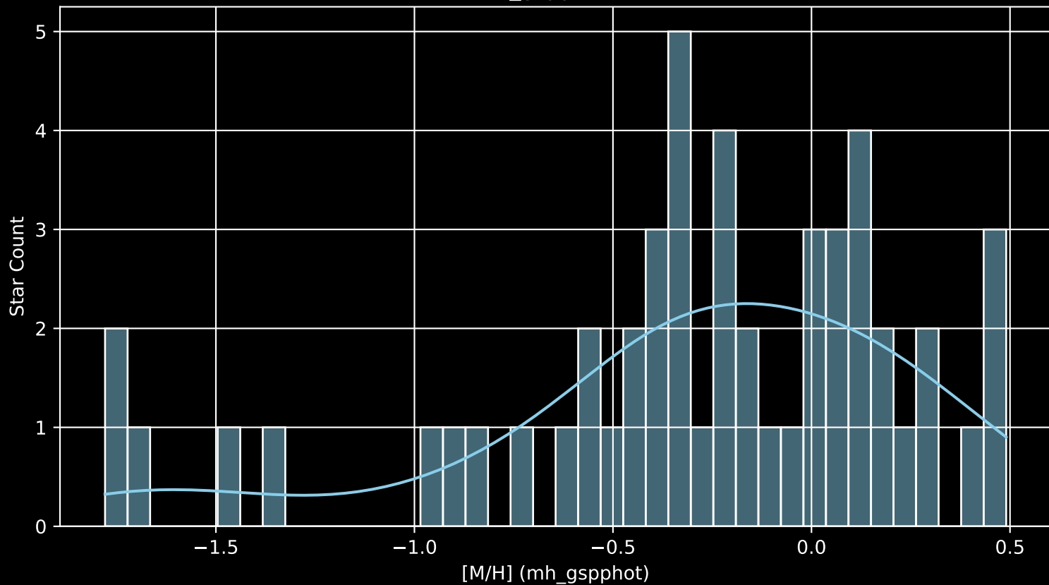
APOGEE DR17 Field: [282-32-O [M/H] (mh_gspphot) (n= 51)
